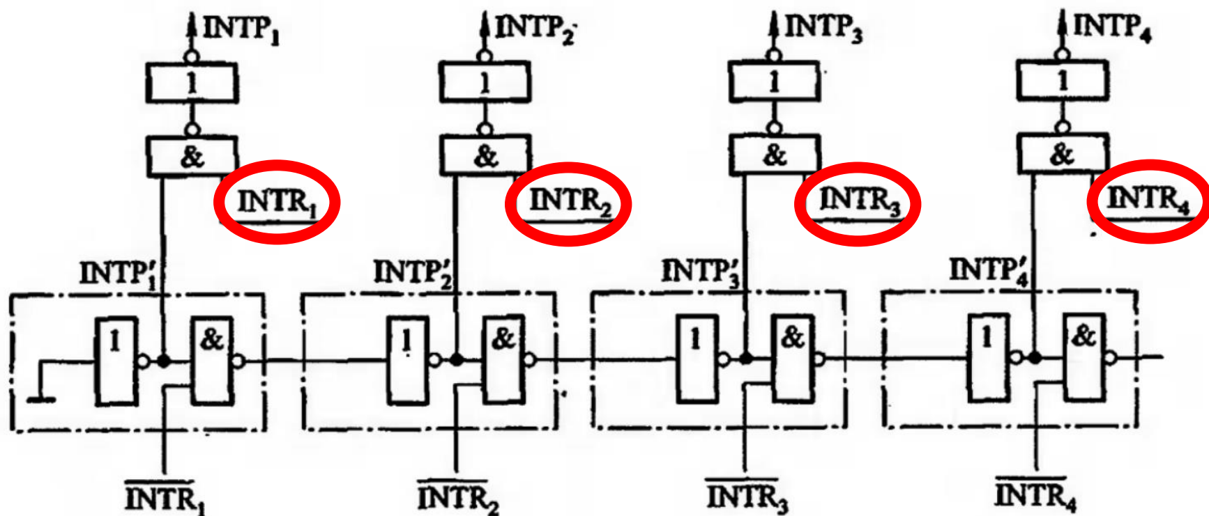
图 5.38 链式排队器
